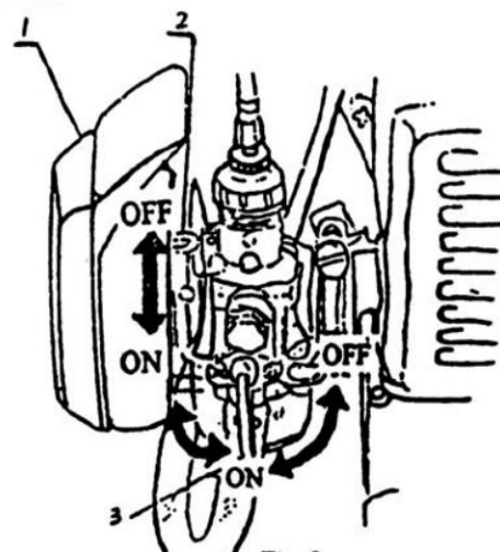
1. Filtro de aire 2. Estrangulador 3. Llave de combustible
